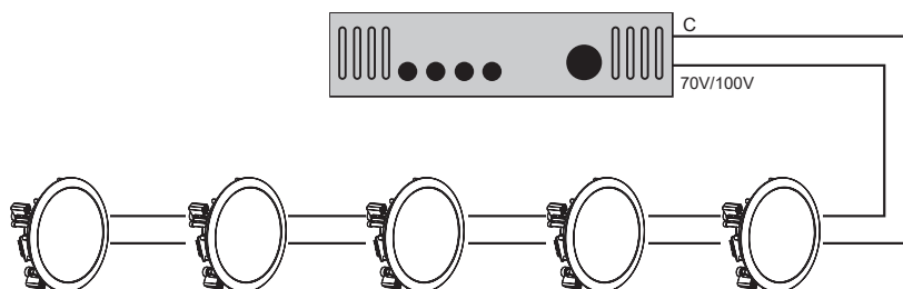
5 altoparlanti collegati in parallelo con terminale del trasformatore a 20W.
