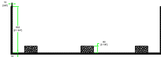
A-A VIEW
